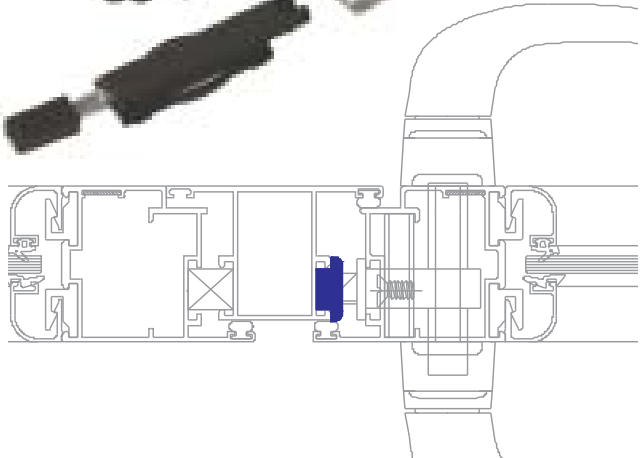
Pestillo cámara europea H-49
