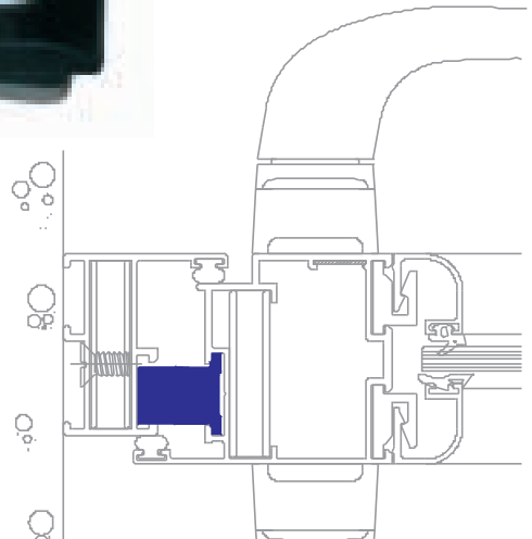
Resbalón cámara europea
