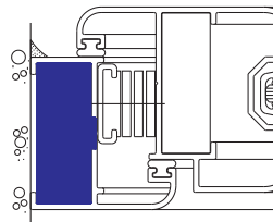
Escuadra 0203 Marco Perfil 4411
