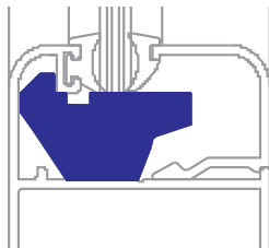
Calzo Paño fijo
