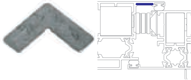
Escuadra de alineamiento 040
