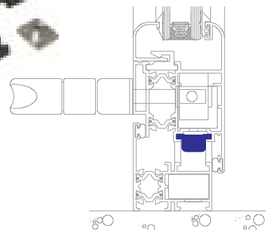
Picaporte camara europea H-49
