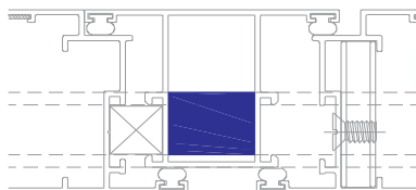
Soportes en "T" Perfil 4434 medida 13,8
