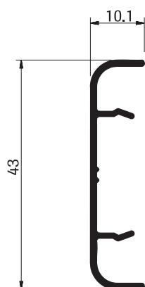
4459 CONTRAMARCO Peso: 0.224 kg/M Espesor: 1.2 mm
