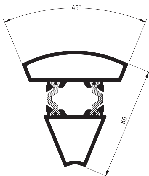
0286 OCTAVO RODON RPT 50 MM. Peso: 0.912 kg/M Espesor: 1.5 mm
