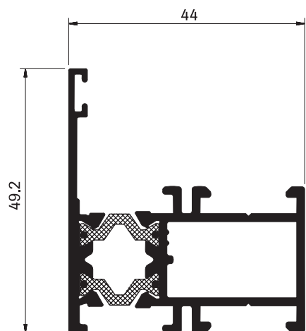
4481 MARCO Peso: 0.919 kg/M Espesor: 1.5 mm
