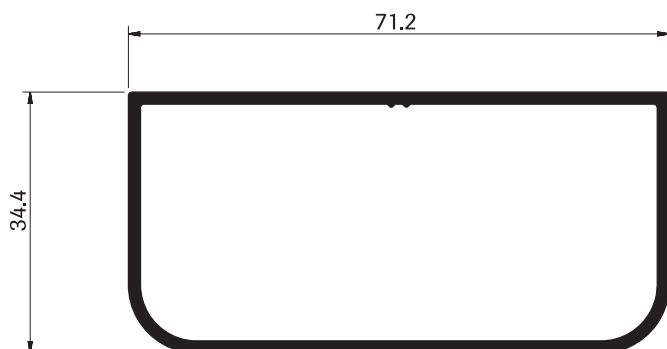
4468 PILAR Peso: 0.854 kg/M Espesor: 1.6 mm
