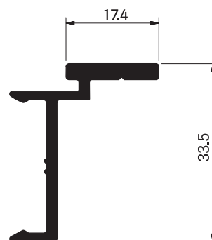
4460 PREMARCO Peso: 0.390 kg/M Espesor: 2.0 mm
