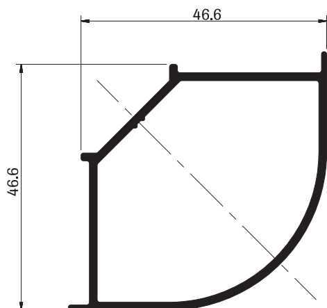
4467 PILAR RODON 90° Peso: 0.656 kg/M Espesor: 1.5 mm
